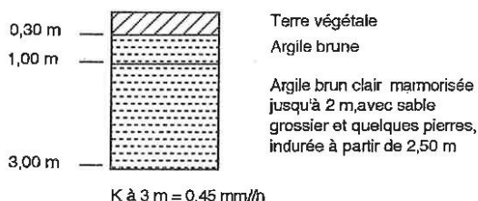
SONDAGE N° 43
