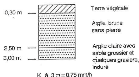
SONDAGE N° 30
