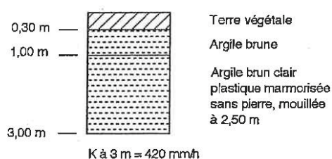
SONDAGE N° 38
