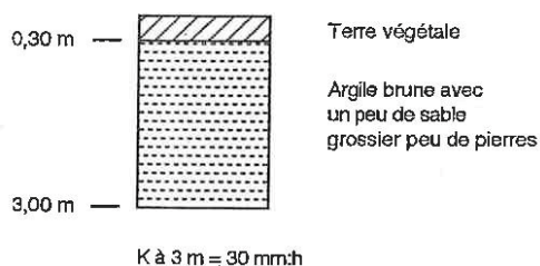
SONDAGE N° 37
