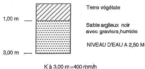
SONDAGE N° 38
