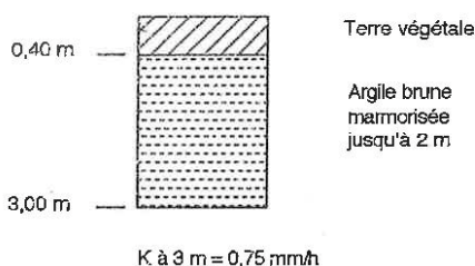
SONDAGE N° 43
