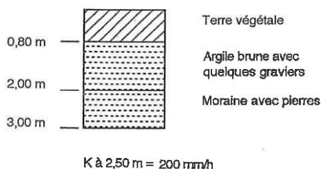
SONDAGE N° 9
