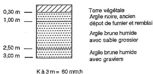
SONDAGE N° 33
