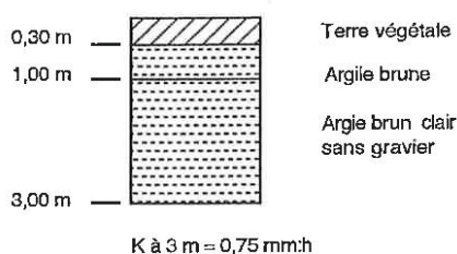
SONDAGE N° 31
