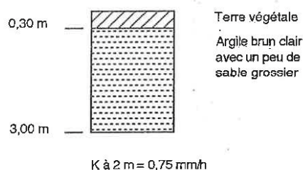
SONDAGE N° 44
