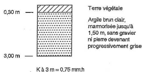
SONDAGE N° 40
