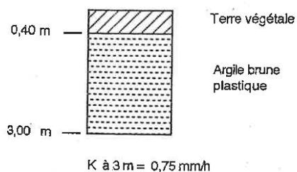
SONDAGE N° 39
