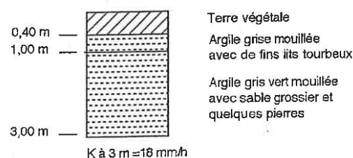
SONDAGE N° 34
