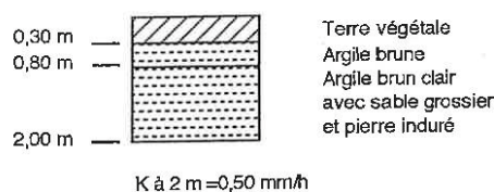
SONDAGE N° 32
