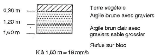
SONDAGE N° 35
