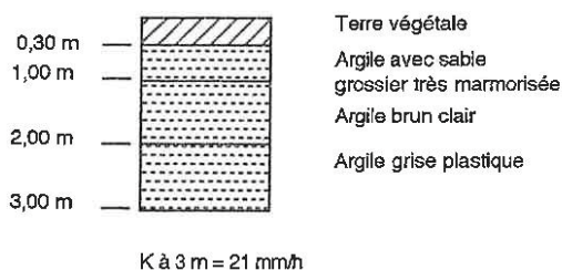
SONDAGE N° 45
