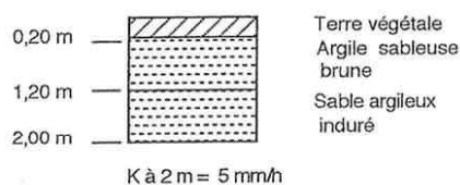
SONDAGE N° 8
