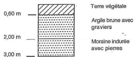
SONDAGE N° 10
