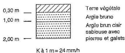
SONDAGE N° 29
